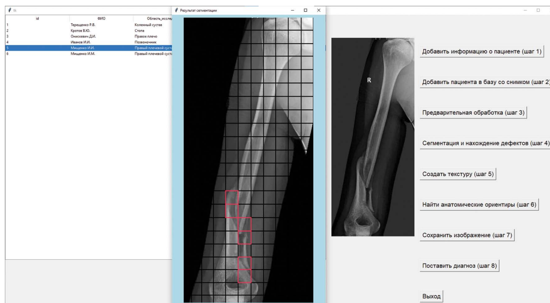
Результат сегментации
