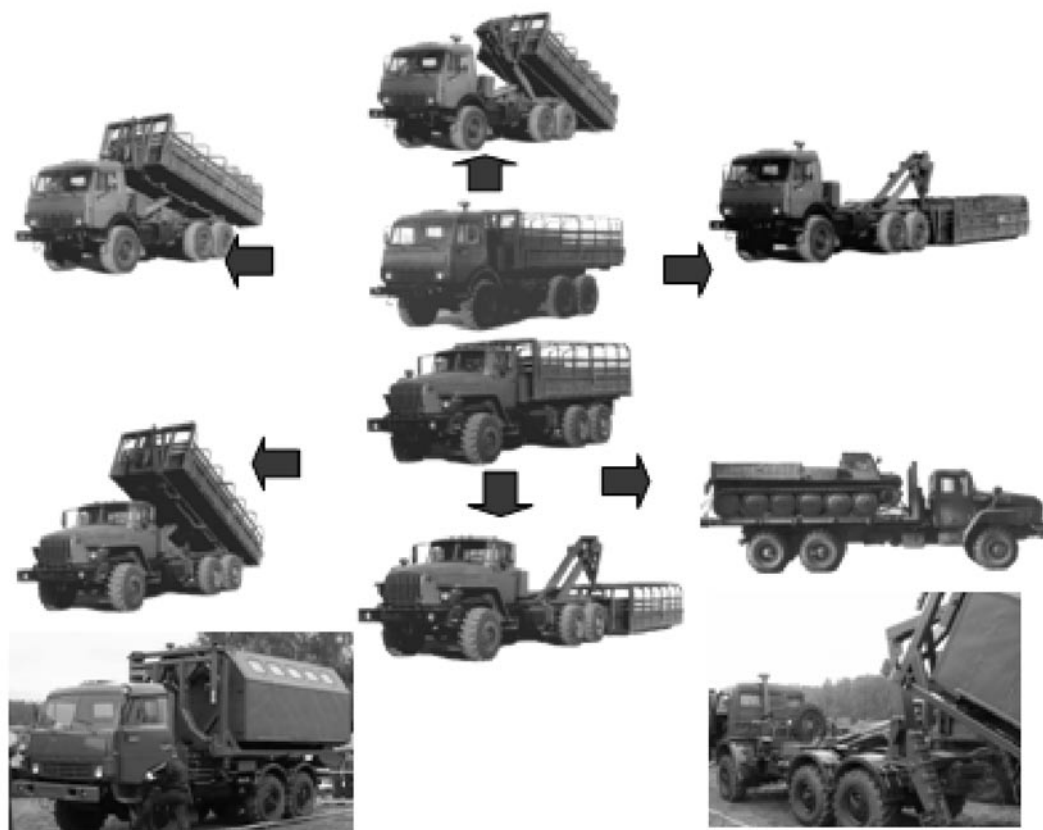
Рис. 3. Макетные образцы системы «Мультилифт» на автомобилях КамАЗ и Урал
